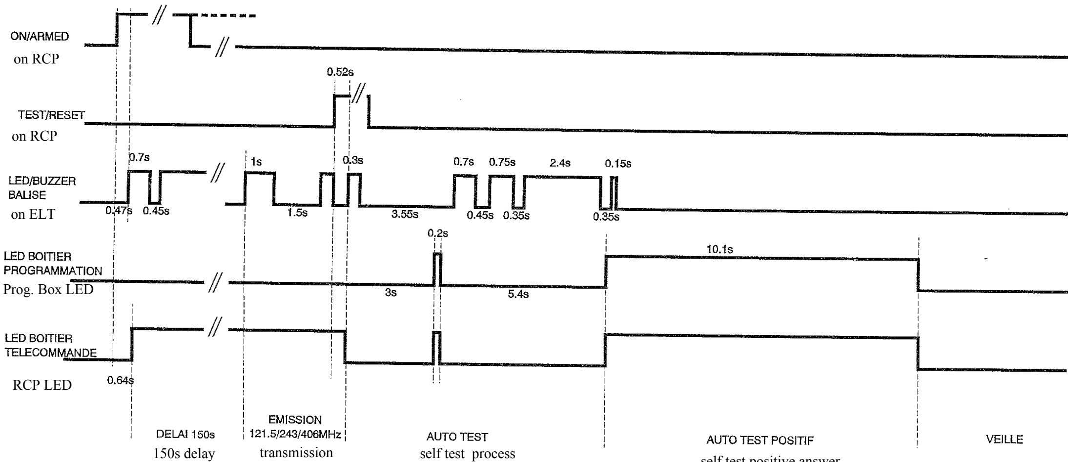
CHRONOGRAMME DU FONCTIONNEMENT DE LA BALISE A06V2, DU BOITIER DE PROGRAMMATION ET DU BOITIER DE TELECOMMANDE Timing diagram for ELT model A06V2 TX, Prog. Box and RCP (Remote Control Panel)
